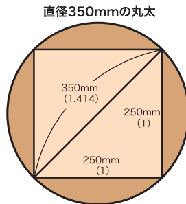
丸太から切り出される正四角柱の寸法
